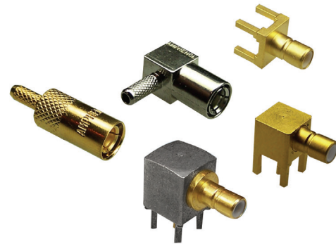
Mini 75 \Omega SMB
