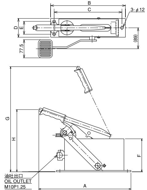
補助レバー使用時 WHEN EXTENSION LEVER USED.
