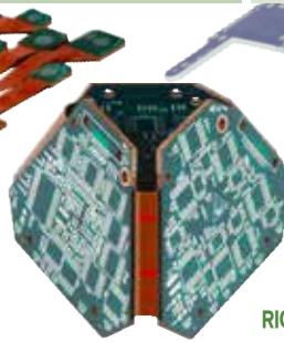
FLEX & RIGID FLEX
