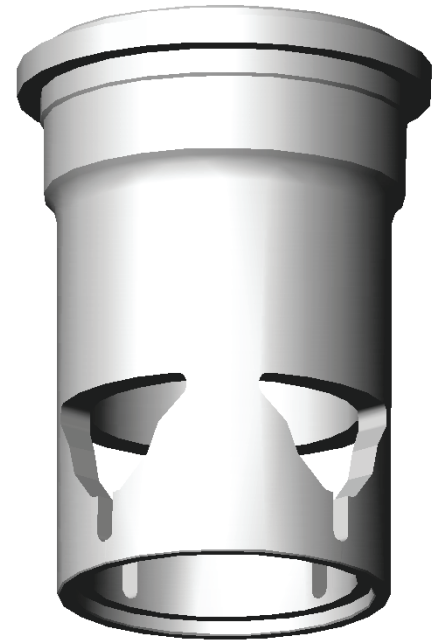
Cage V-Port
