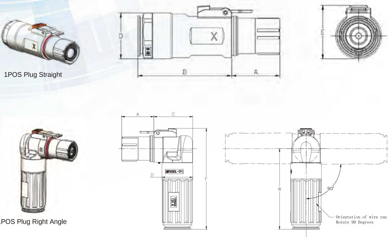
PowerLok™ 1POS Assembly Plug Connector Parameter
