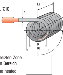
Vorrichtung zum Wendeln Coiling fixture
