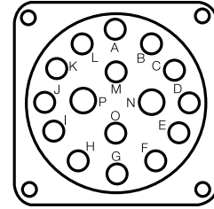
MOTOR CONNECTOR MS3102E-24-07P
