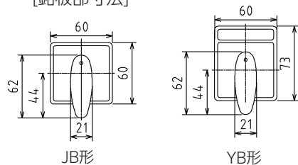
[取付寸法]
