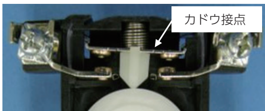
銀ツイン、金ツイン接点
