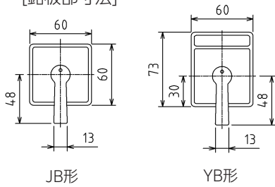
[取付寸法]
