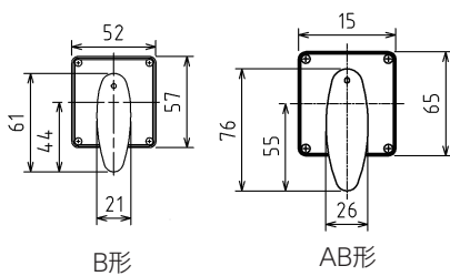
[銘板部寸法]
