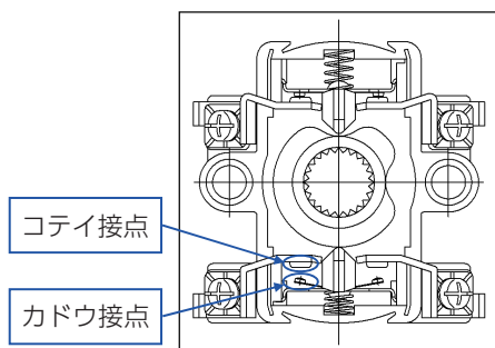
標準（銀シングル）接点
