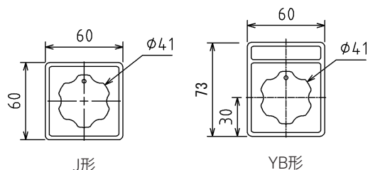
[取付寸法]
