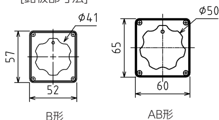
[取付寸法]
