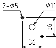
[取付寸法]
