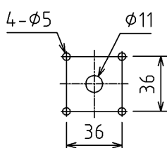
[取付寸法]
