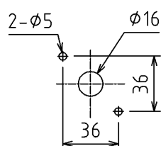
[取付寸法]
