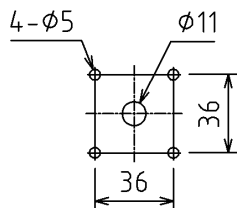
[取付寸法]
