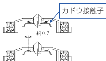
接点のワイプ構造
