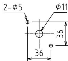
[取付寸法]
