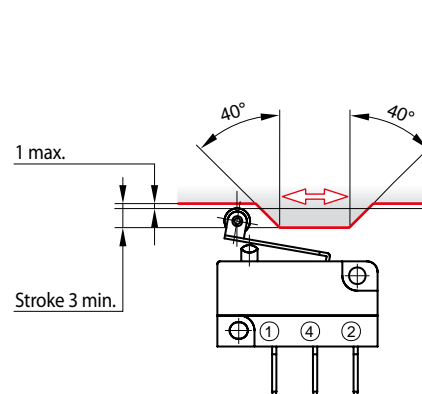
Linear cam
